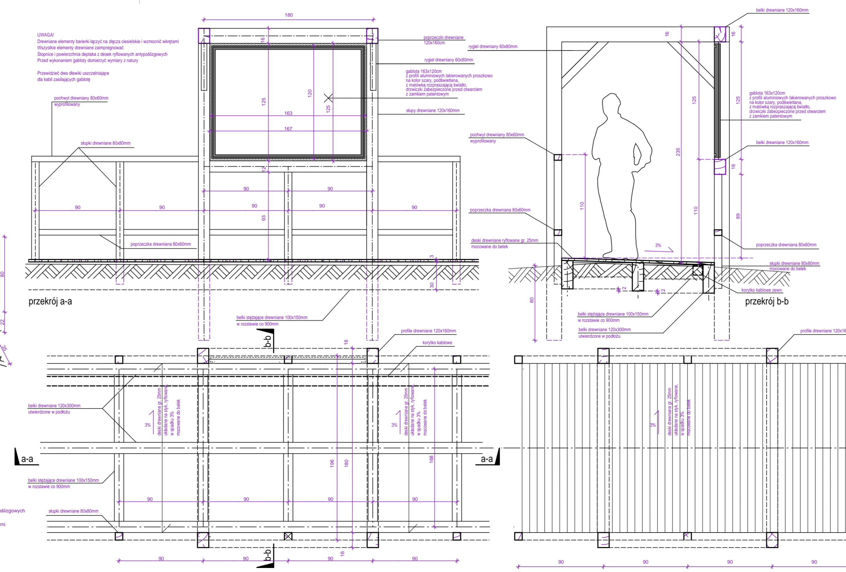
gablota wystawowa, detal skala 1:25
