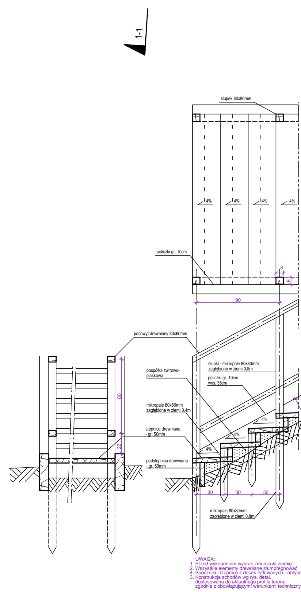
schody, detal skala 1:25
